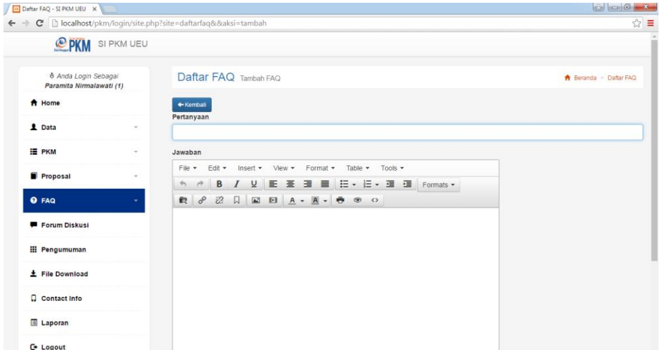
Gambar 25 Halaman Menambah FAQ
